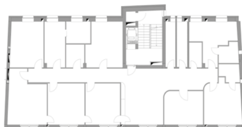
Beispielgrundriss, 2. OG, verzimmert
